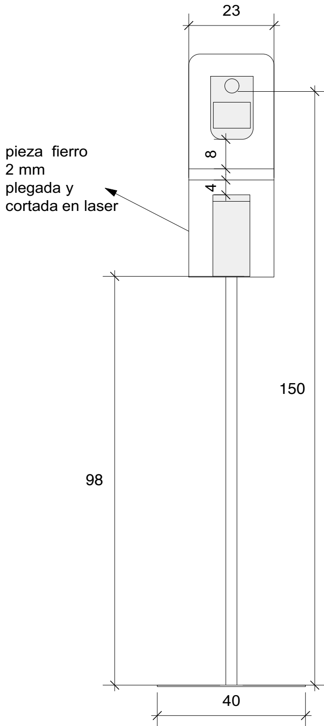
Elevacion frontal
